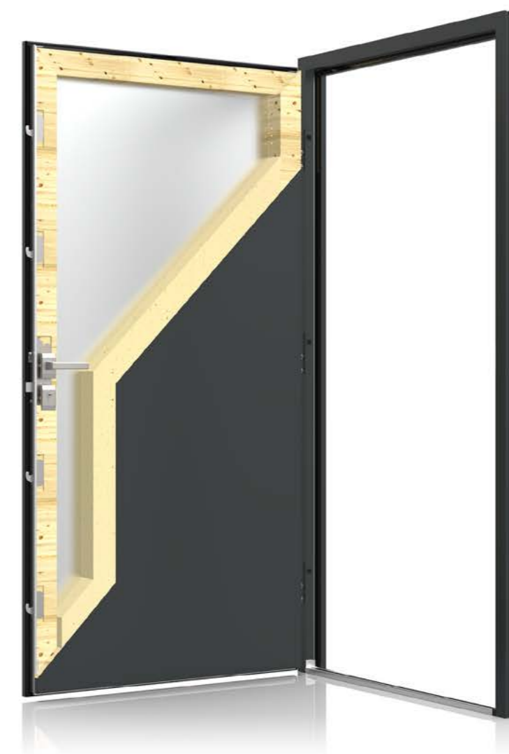
Zamek listwowy: 5 punktowy hakowy lub 3 punktowy automatyczny
